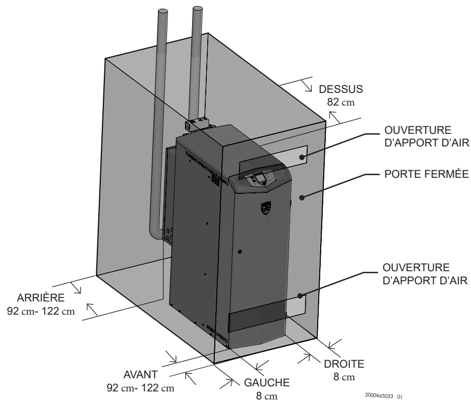
Figure 1-2 Distances de dégagement minimales - Garde-robe
