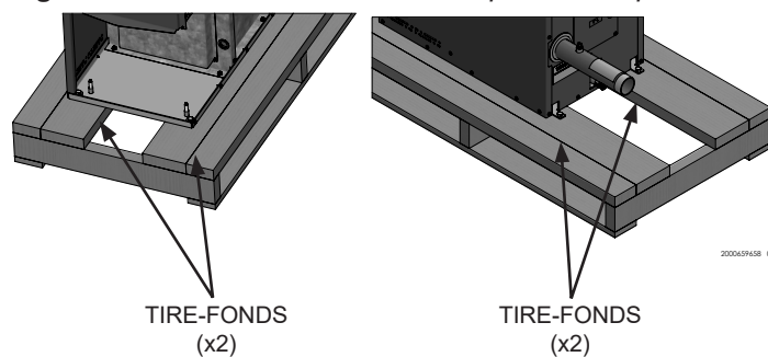
Figure 2-1 Chaudière montée sur sa palette d'expédition
