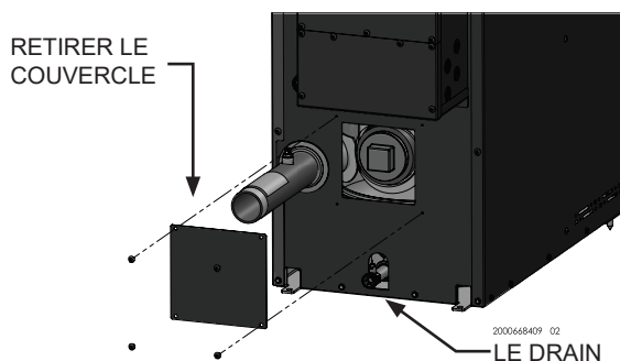
Figure 7-1 Retirer le couvercle d'inspection
