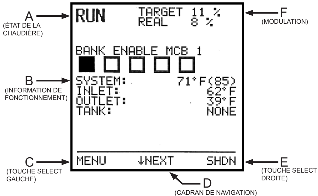
Figure 6-2 Écran d'affichage de l'état
