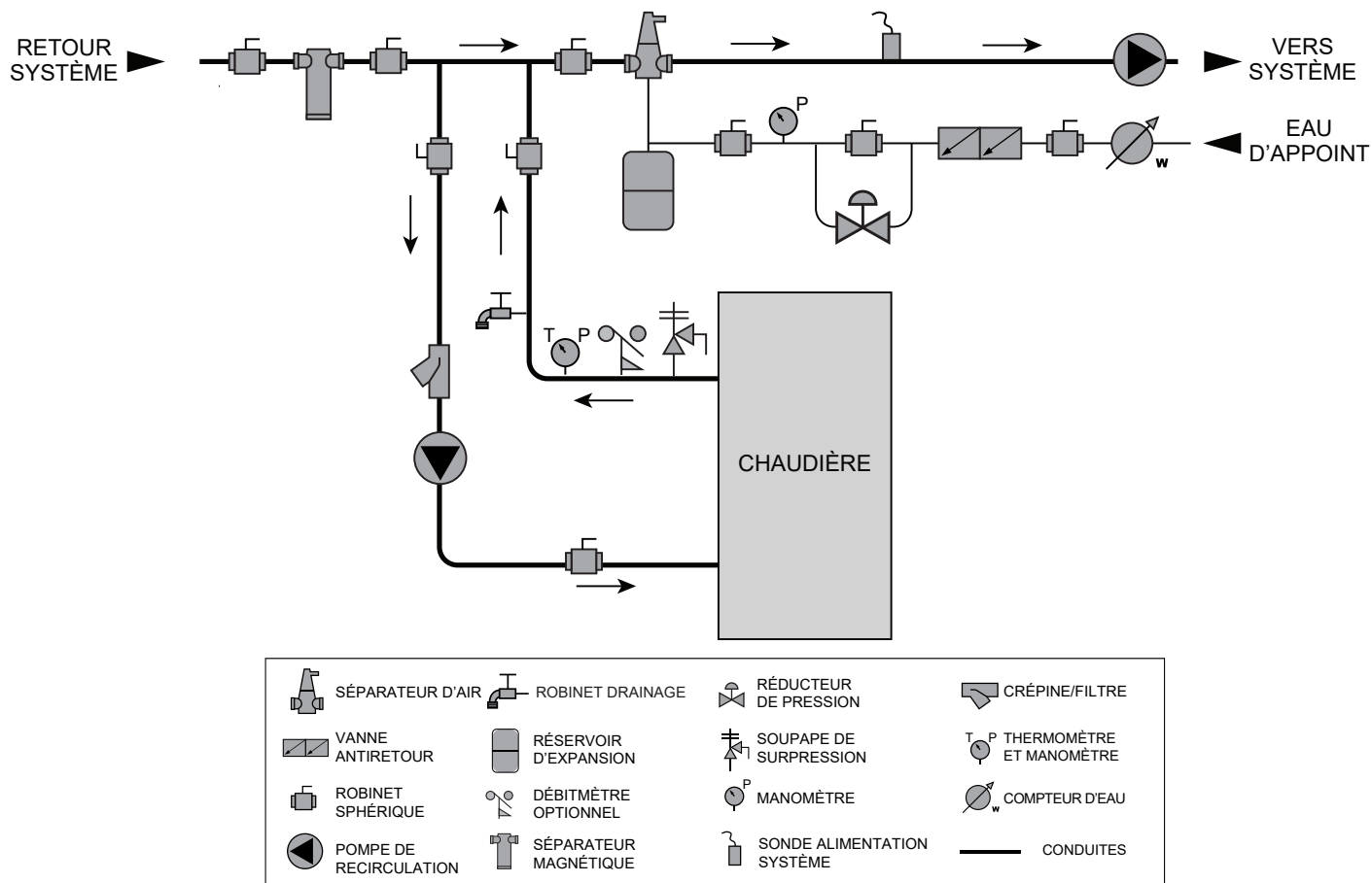
Figure 3-2A Tuyauterie à proximité de la chaudière avec raccord en Y
