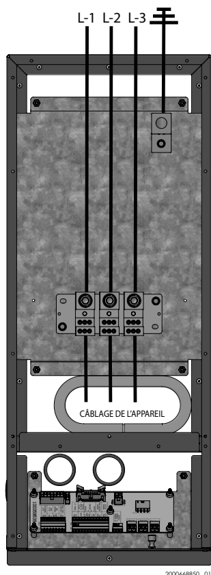
Figure 4-1 Raccords basse tension au chantier
