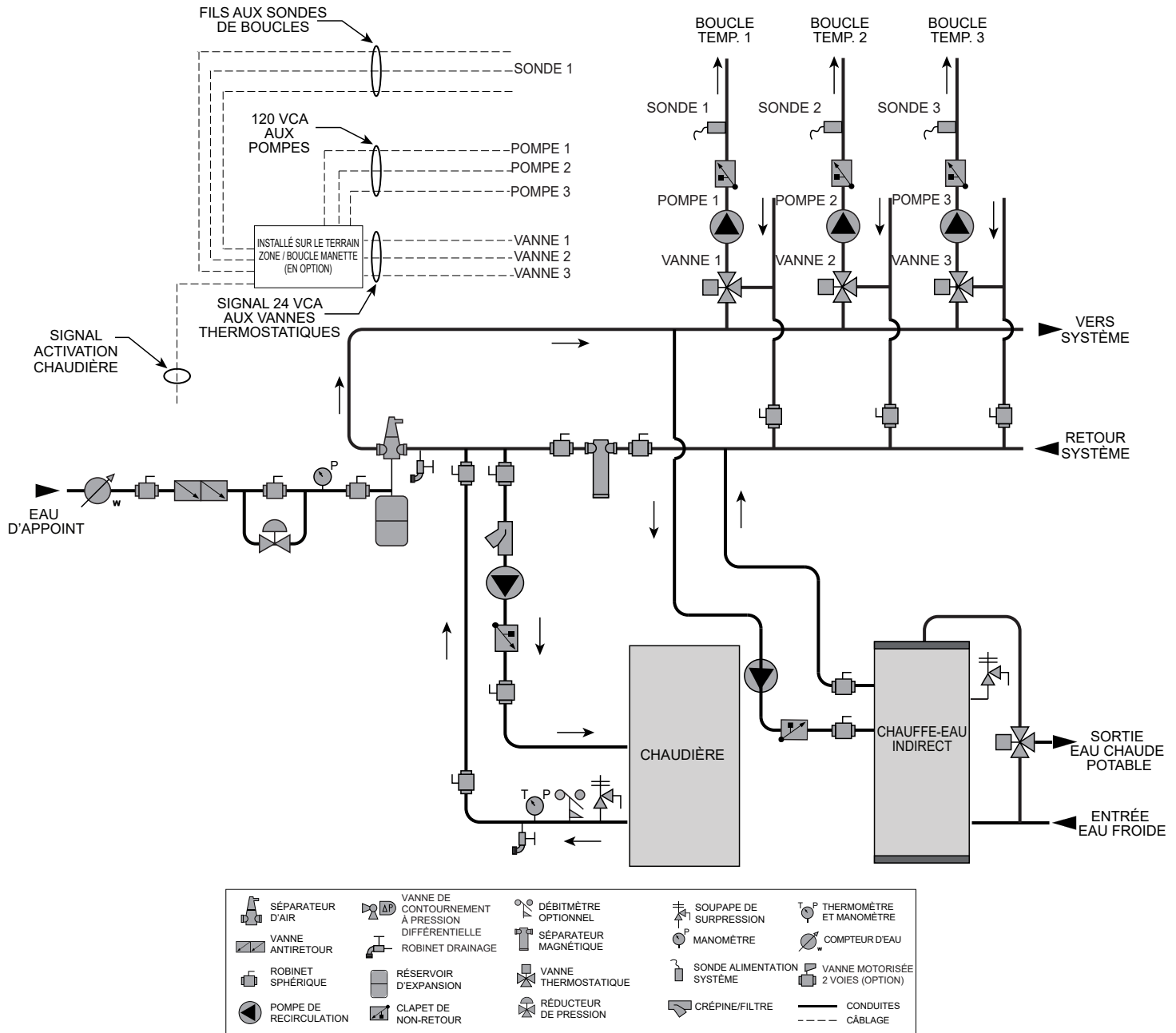
Figure 3-9 Chaudière unique - Multitempérature avec eau potable comme zone distincte
