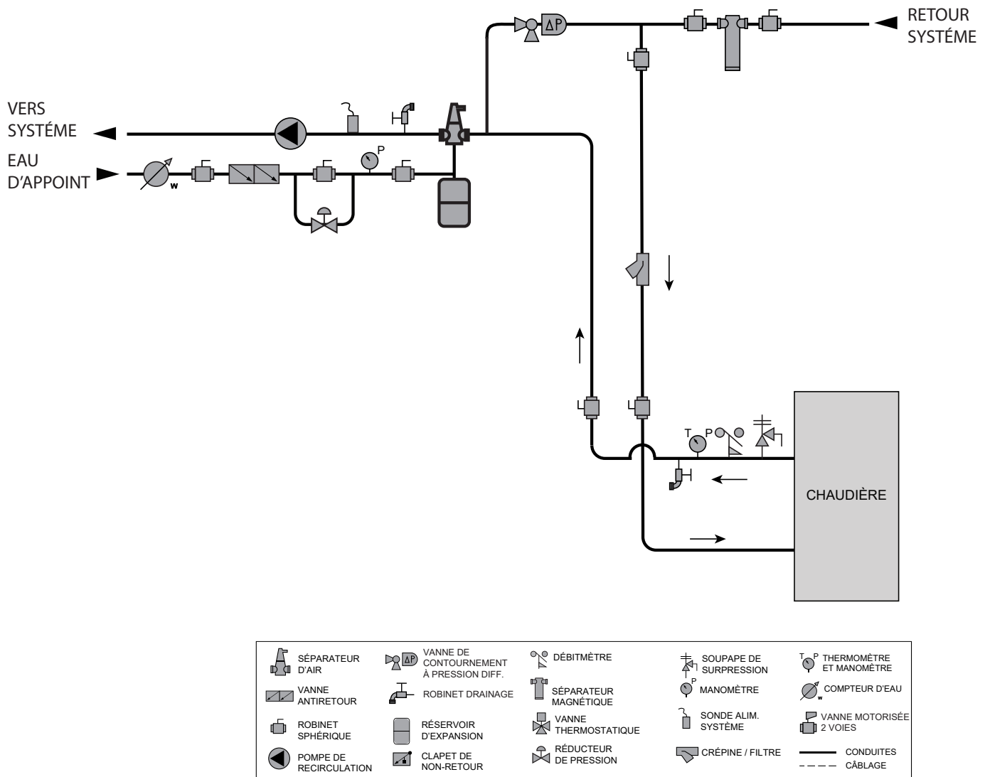
Figure 3-2C Tuyauterie à proximité de la chaudière avec collecteur à faible perte
