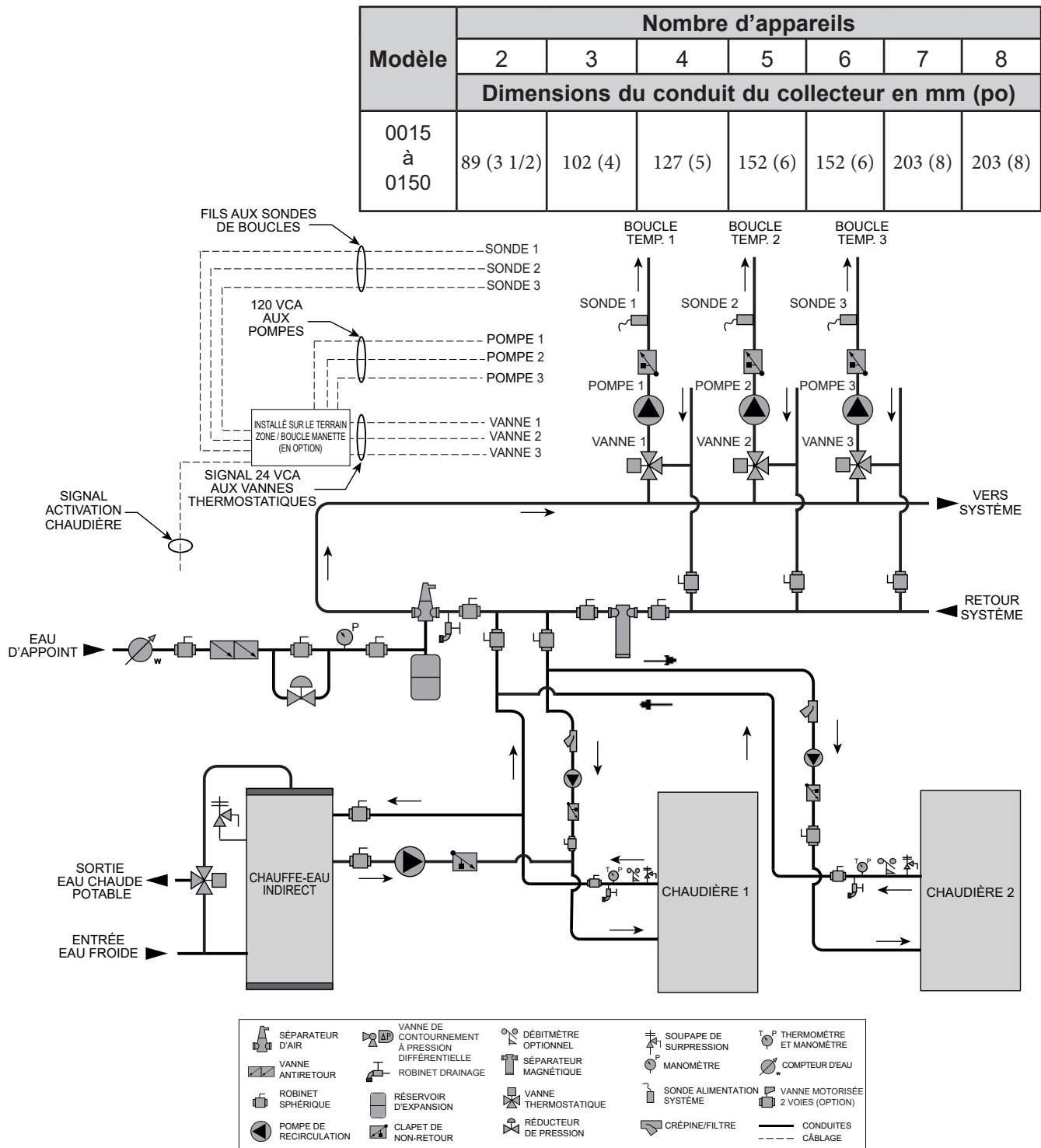
Figure 3-7 Plusieurs chaudières - Multitempérature
