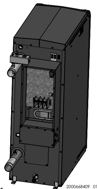
Figure 4-2 Acheminement du câblage réalisé sur les lieux
