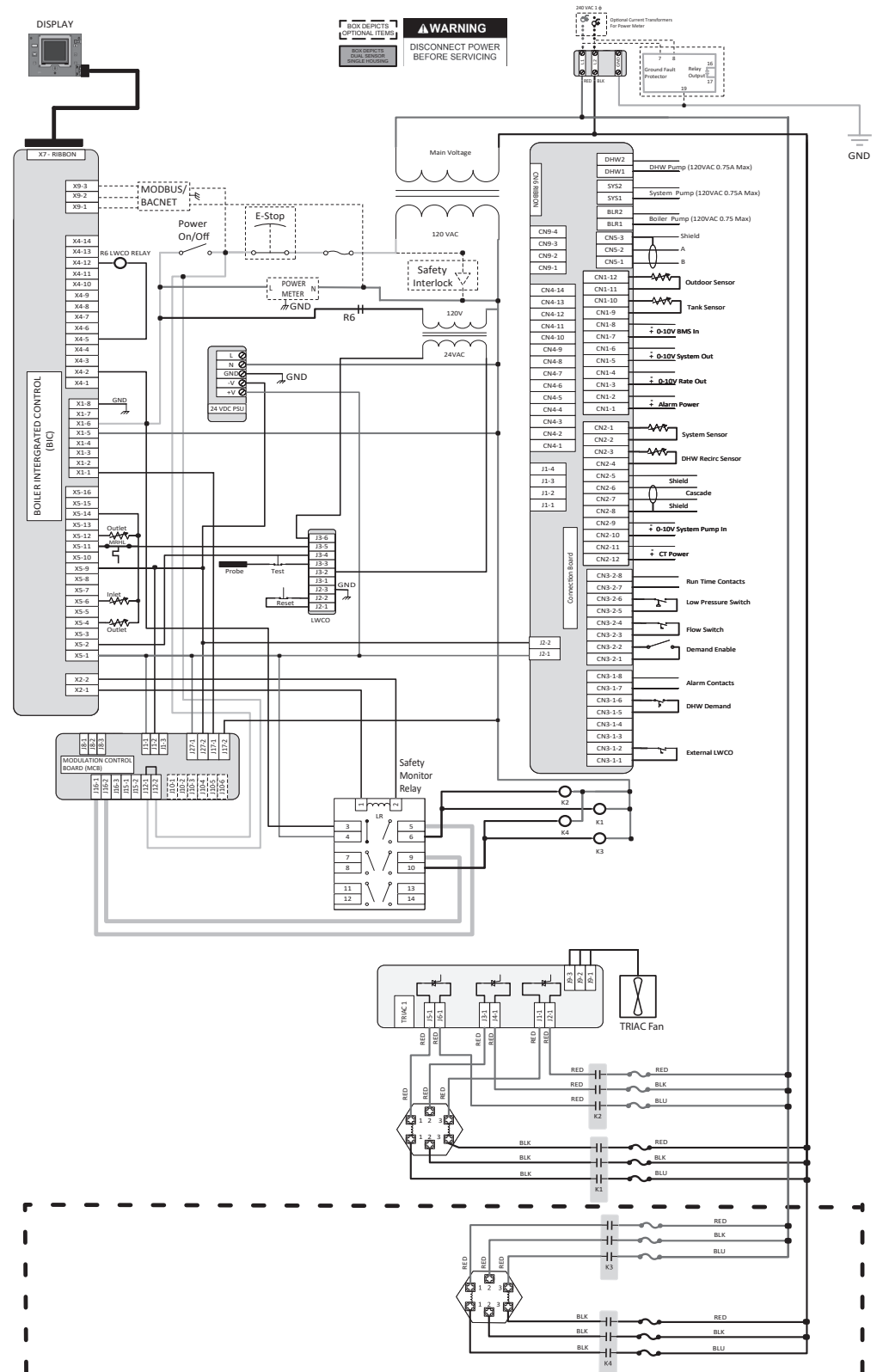
Figure 8-8 Schéma électrique - 240V, 1 Phase (A)
