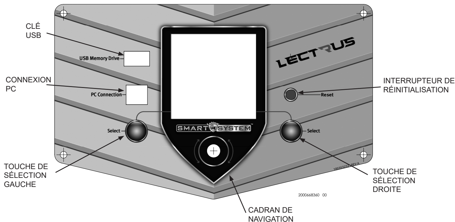
Figure 6-1 Module de commande
