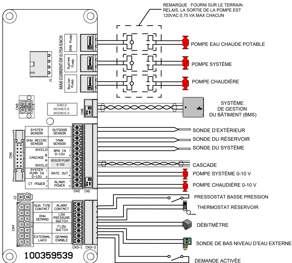
Figure 4-3 Raccords de tension au chantier
