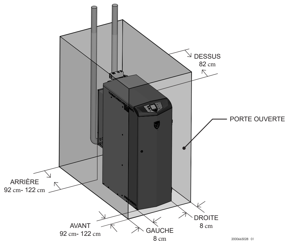
Figure 1-1 Distances de dégagement minimales - Alcôve
