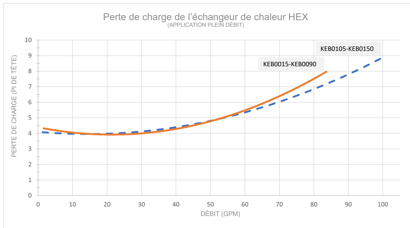
Figure 3-3 Perte de charge par rapport au débit
