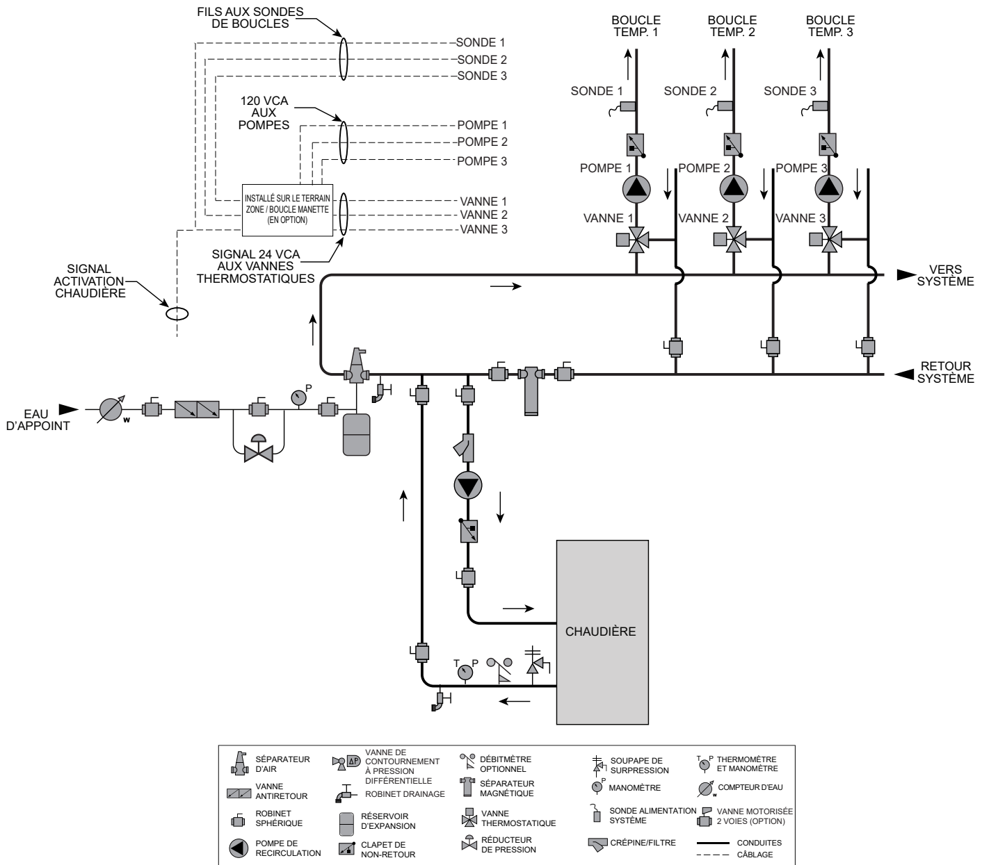
Figure 3-5 Chaudière unique - Multitempérature
