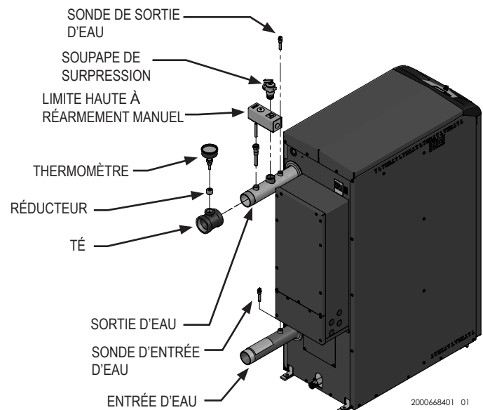
Figure 3-1 Installation de jauge T&P - Modèles 0015 - 0150
