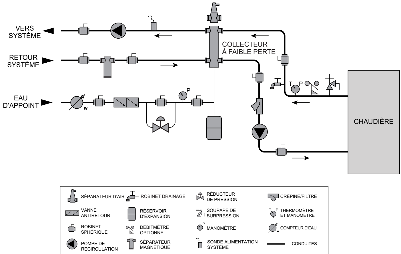
Figure 3-2B Tuyauterie à proximité de la chaudière avec collecteur à faible perte
